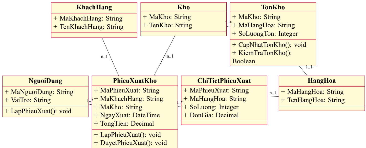
Hình 4.6: Biểu đồ lớp trong ca sử dụng UC10 – Lập phiếu xuất kho
