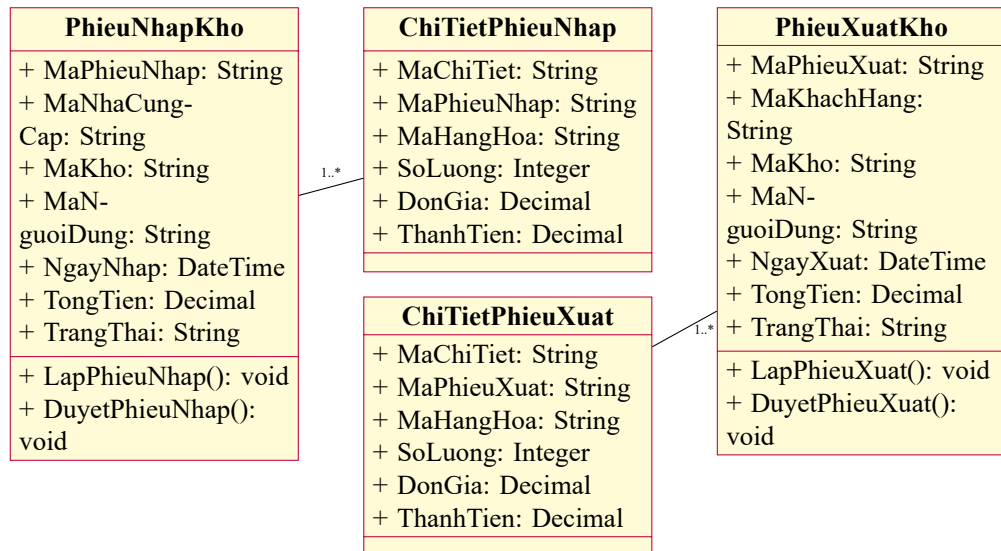
Hình 4.2: Sơ đồ lớp nghiệp vụ nhập xuất kho
