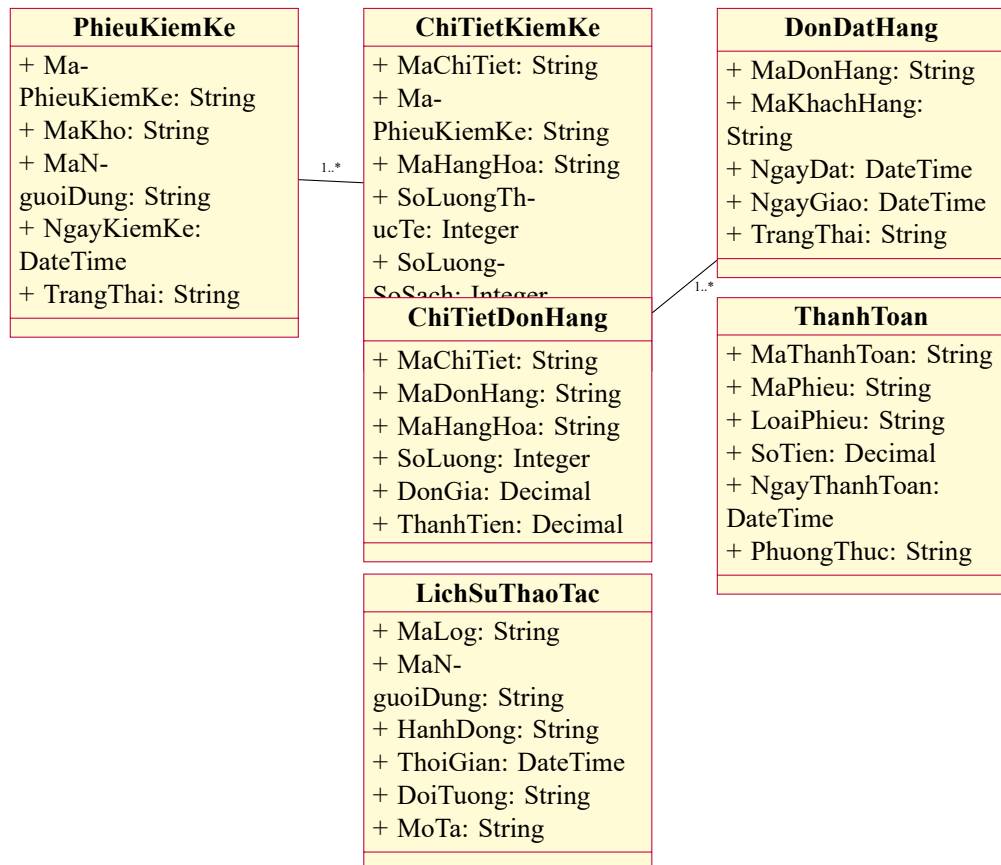
Hình 4.3: Sơ đồ lớp kiểm kê, đơn hàng và thanh toán
