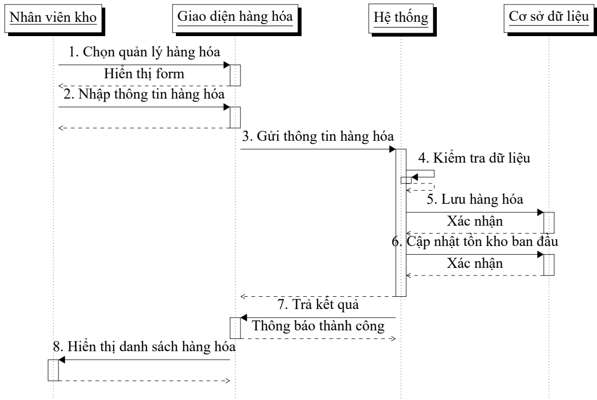
Hình 5.1: Sequence diagram UC05 – Quản lý hàng hóa
