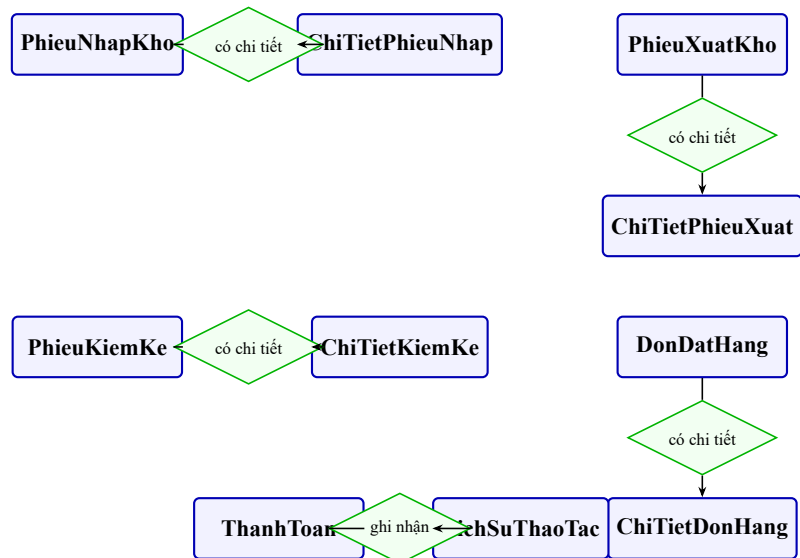
Hình 7.2: Sơ đồ ERD – Nghiệp vụ (Transaction)
