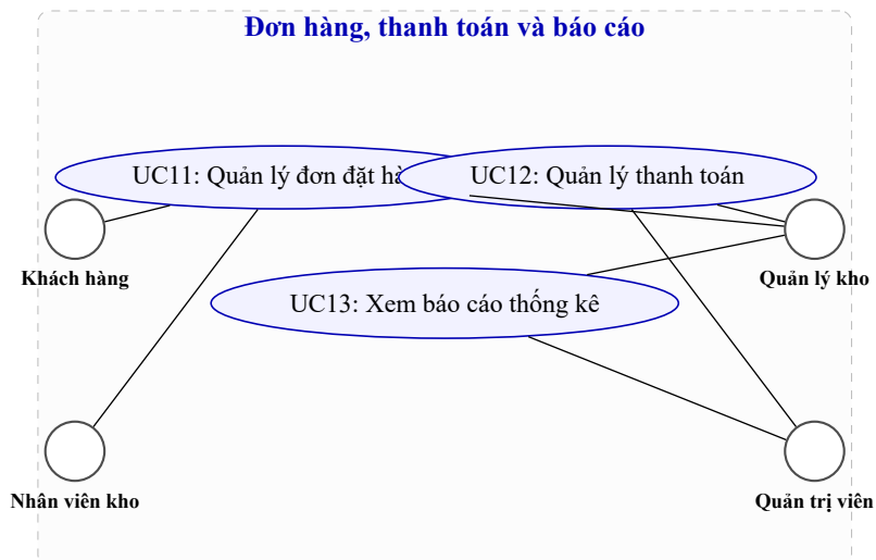
Hình 3.9: Sơ đồ use case phân rã – Đơn hàng, thanh toán và báo cáo
