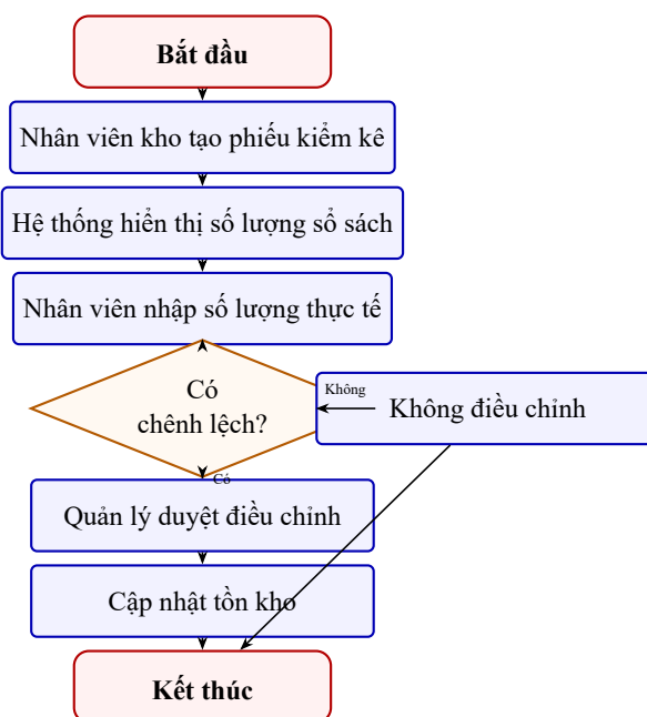
Hình 2.3: Sơ đồ hoạt động quy trình kiểm kê tồn kho
