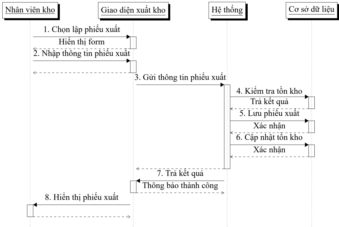
Hình 5.4: Sequence diagram UC10 – Lập phiếu xuất kho
