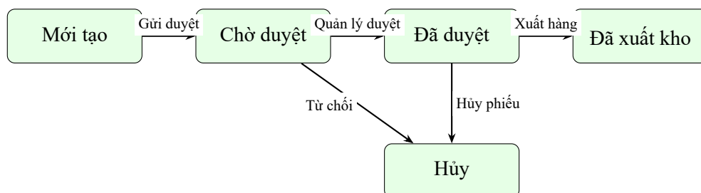
Hình 5.6: State Machine Diagram – Trạng thái phiếu xuất kho
