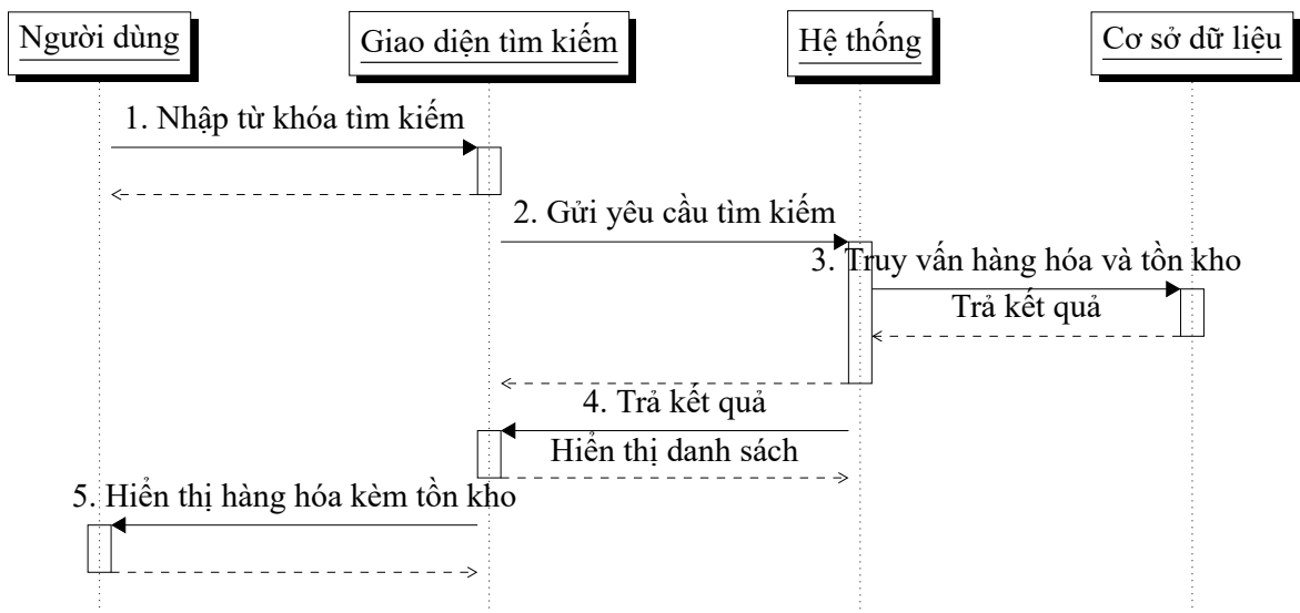
Hình 5.2: Sequence diagram UC06 – Tìm kiếm hàng hóa
