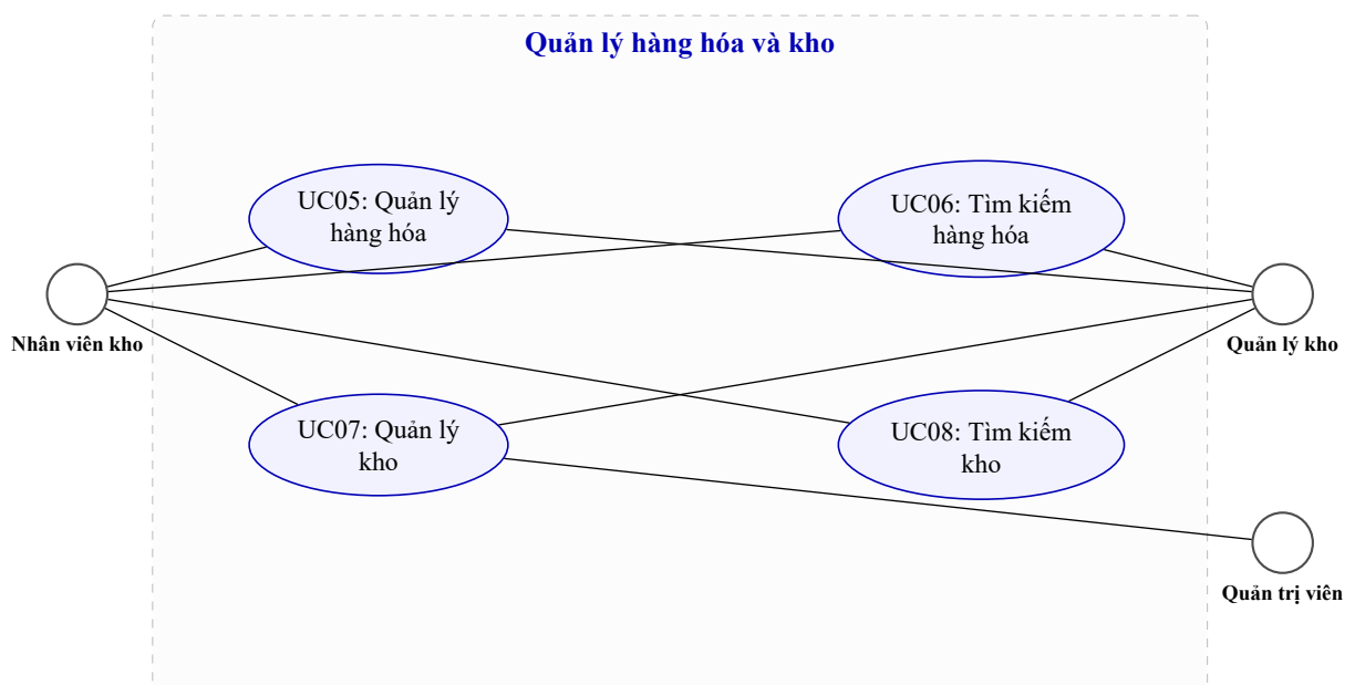
Hình 3.7: Sơ đồ use case phân rã – Quản lý hàng hóa và kho
