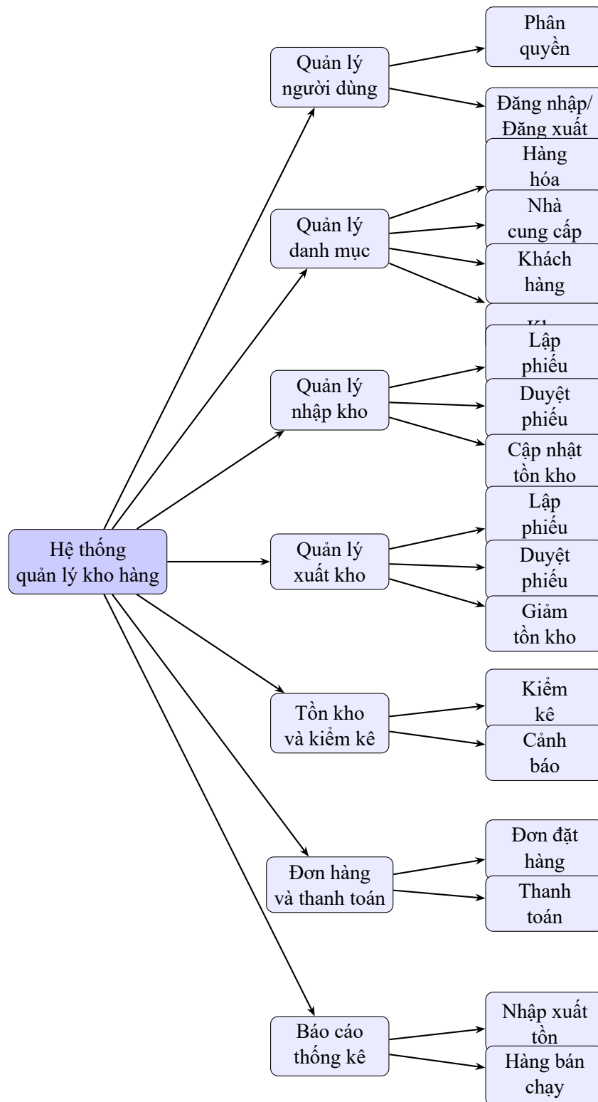
Hình 3.1: Sơ đồ phân cấp chức năng (BFD) hệ thống quản lý kho hàng
