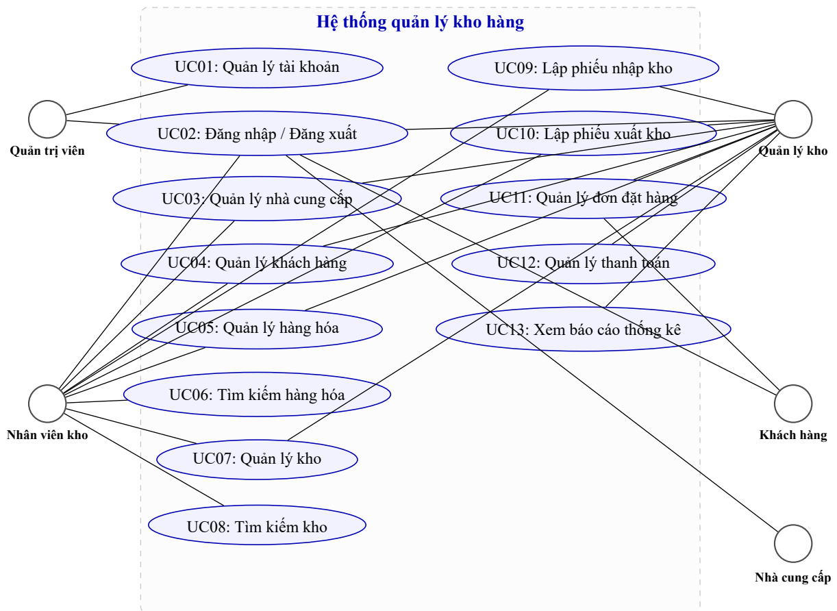
Hình 3.4: Sơ đồ use case tổng quát của hệ thống quản lý kho hàng
