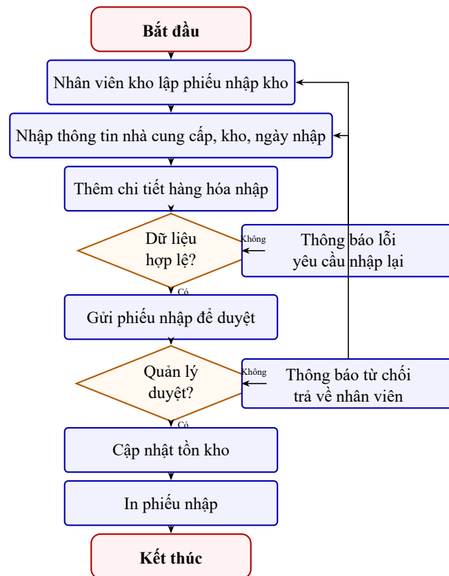
Hình 2.1: Sơ đồ hoạt động quy trình nhập kho
