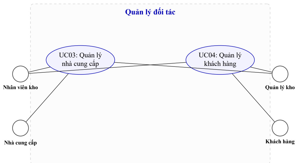
Hình 3.6: Sơ đồ use case phân rã – Quản lý đối tác
