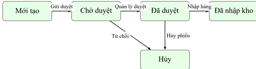
Hình 5.5: State Machine Diagram – Trạng thái phiếu nhập kho
