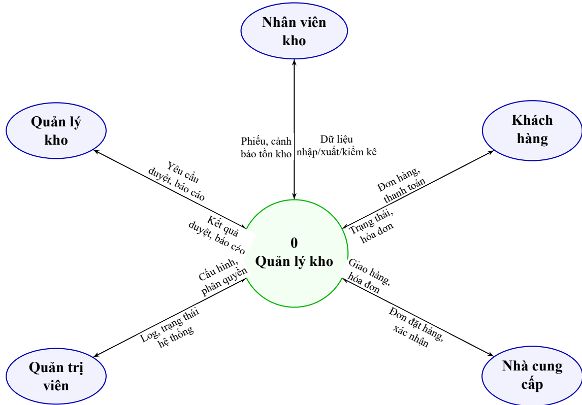
Hình 3.2: DFD cấp 0 (Context Diagram) – Hệ thống quản lý kho hàng
