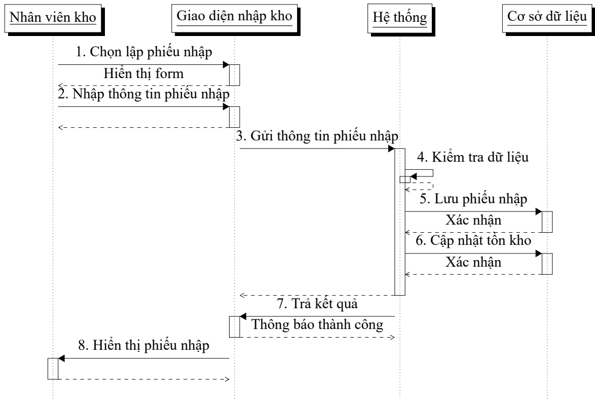
Hình 5.3: Sequence diagram UC09 – Lập phiếu nhập kho
