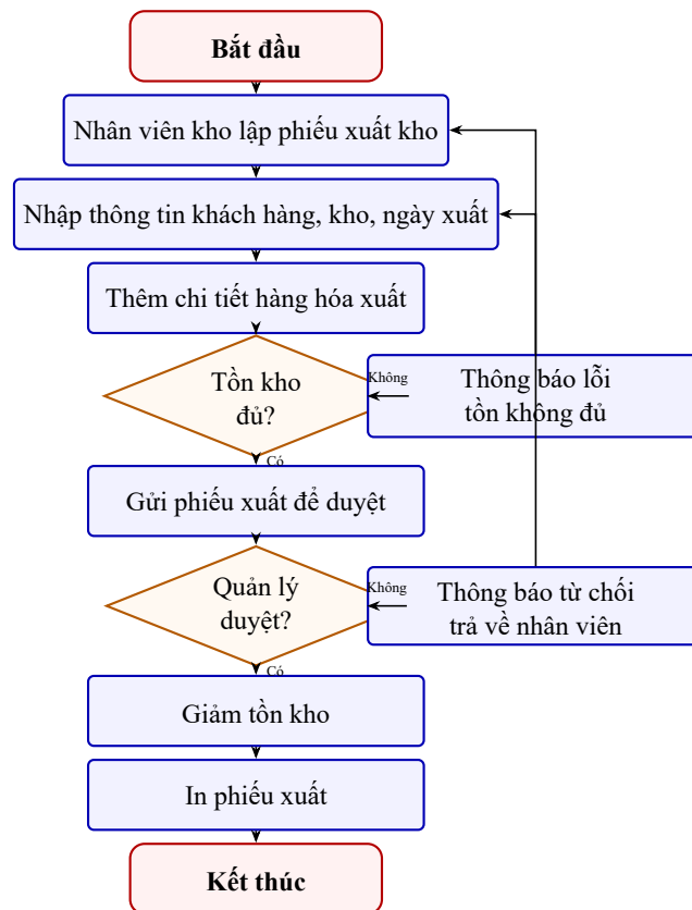
Hình 2.2: Sơ đồ hoạt động quy trình xuất kho
