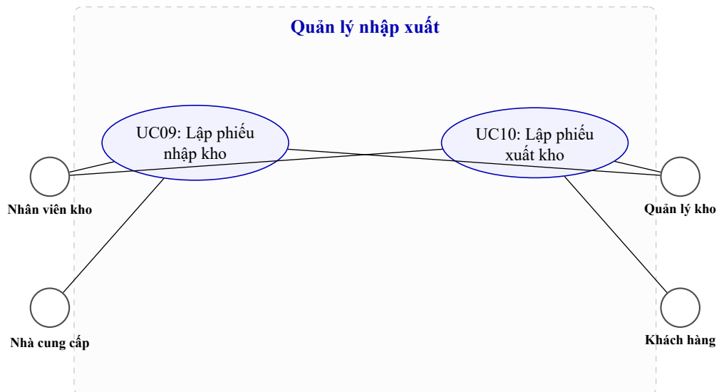
Hình 3.8: Sơ đồ use case phân rã – Quản lý nhập xuất
