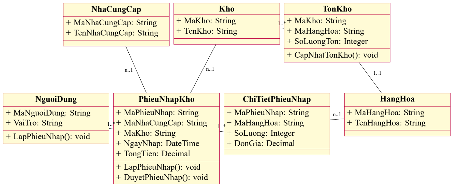
Hình 4.5: Biểu đồ lớp trong ca sử dụng UC09 – Lập phiếu nhập kho
